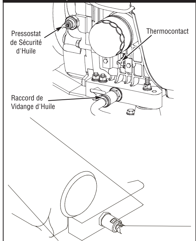
Figure 14 — Faible Pression d'Huile et Température Élevée Interrupteurs
